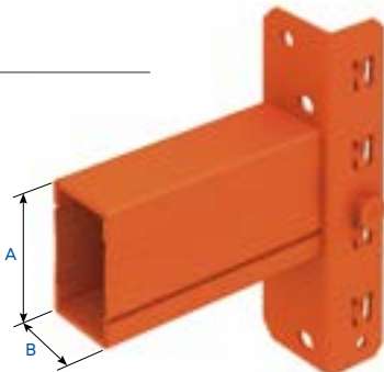
Viga 2C-S (1115) Formada por dois perfis em forma de "C" encaixados um dentro do outro e soldados a um grampo.
