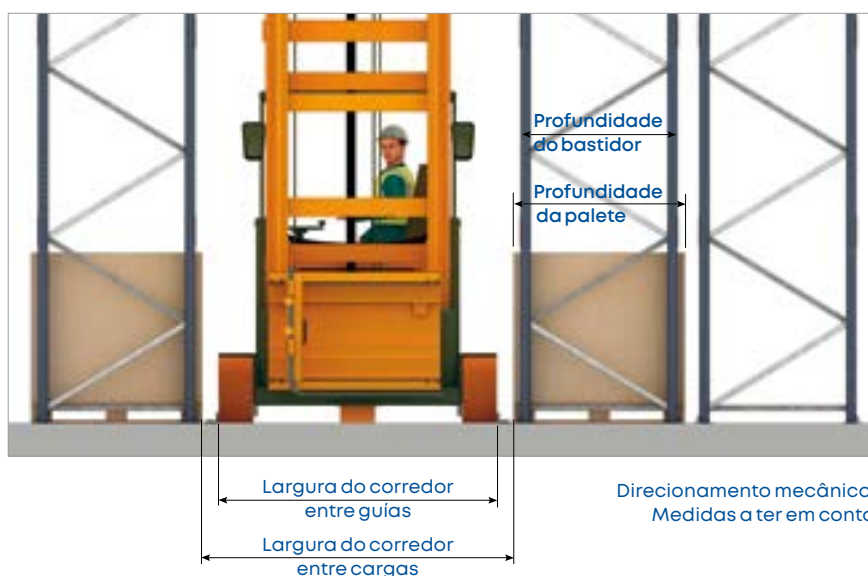
Direcionamento mecânico. Esquema geral
