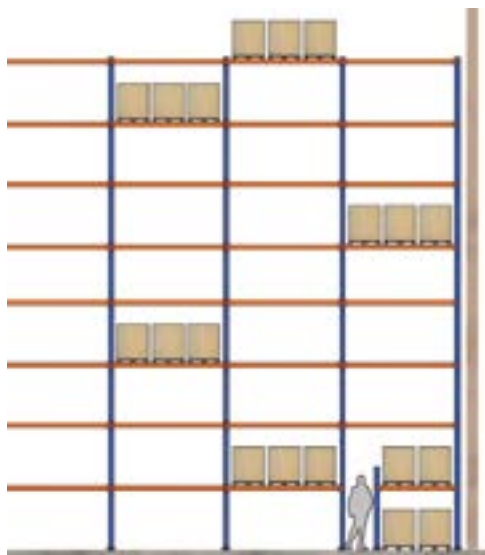
Vista lateral de uma instalação com passagem
