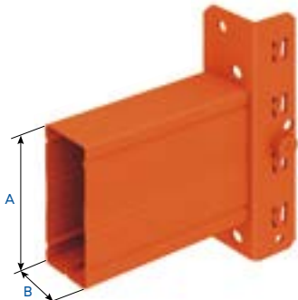
Larguero TB (100, 120, 130)
