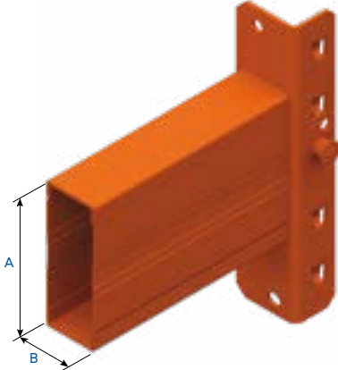
Viga 2C-S (1315, 1515, 1615, 1718) Vigas utilizadas para grandes cargas e comprimentos devido à sua grande resistência.
